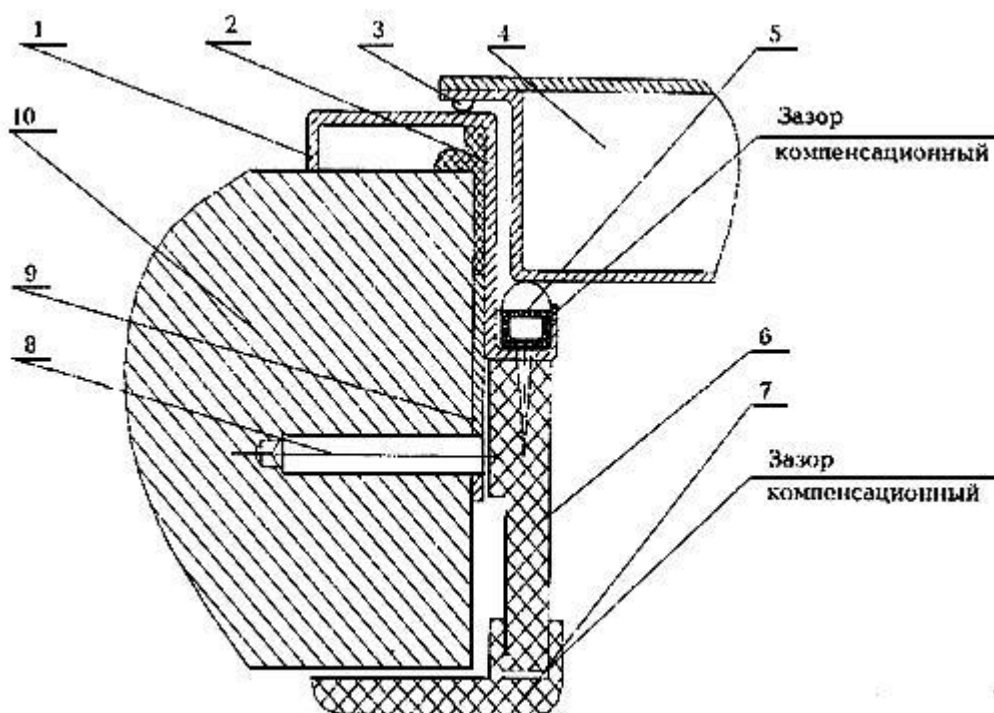
Рисунок Е.1 - Вариант исполнения монтажного узла внутреннего дверного блока
