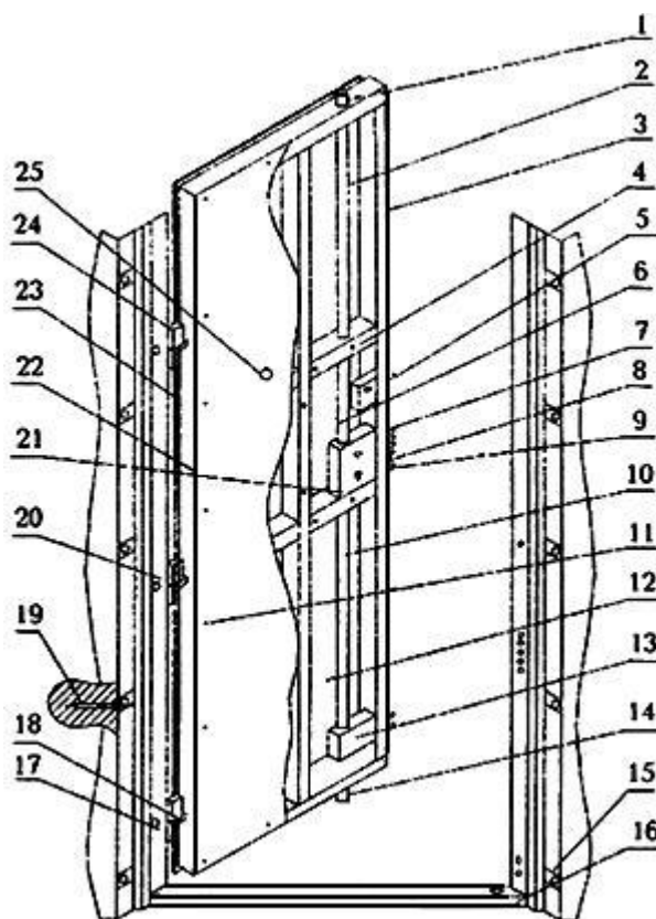
Рисунок 1 - Пример конструкции дверного блока, полотно которого сварено из двух стальных листов и стальных профилей, коробка (рама) - из стального гнутого профиля
