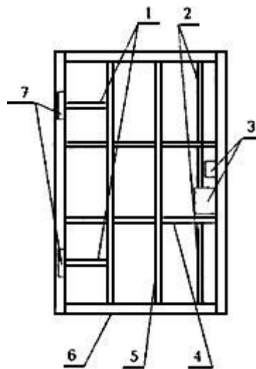
Рисунок 8 - Примеры расположения усиливающих профилей в дверном полотне
