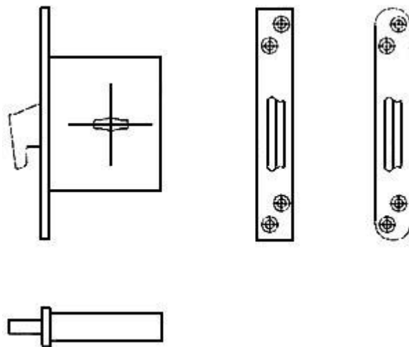
Рисунок Б.4 - Пример замка с крюкообразным засовом
