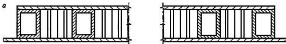
Рисунок 2 - Примеры конструкций дверных полотен
