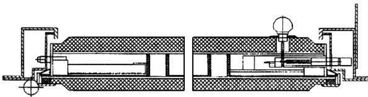
Рисунок 4 - Пример конструкции дверного блока, сваренного из стальных листов и профилей, с облицовкой из натуральной древесины
