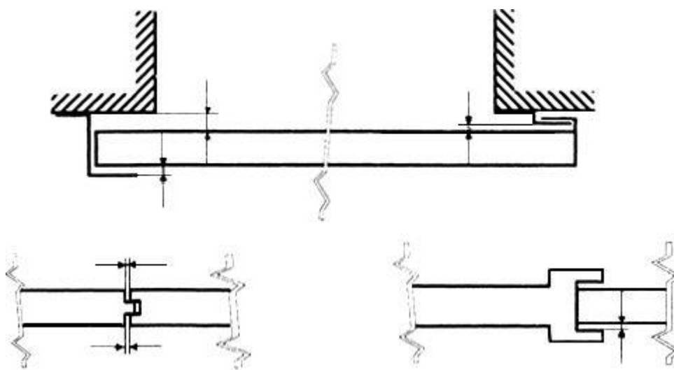
а - откатная дверь (ворота)
