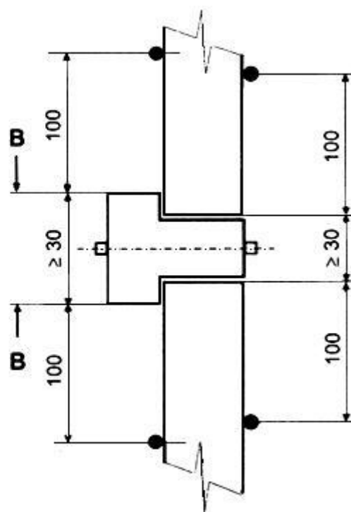
Рисунок 20 - Схема установки термодатчиков на необогреваемой поверхности распашной двупольной двери с фрамугой в зоне 100 мм от торцевых поверхностей коробки (вертикальное сечение)
