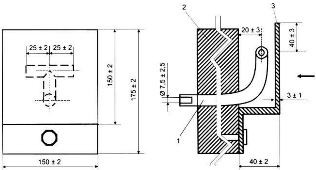
Рисунок 2 - Устройство для измерения давления в печи
