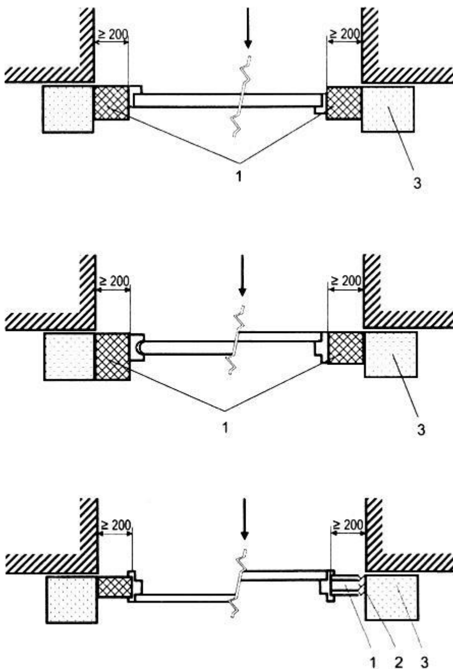
Рисунок 5 - Схемы монтажа образцов распашных дверей (горизонтальное сечение)
