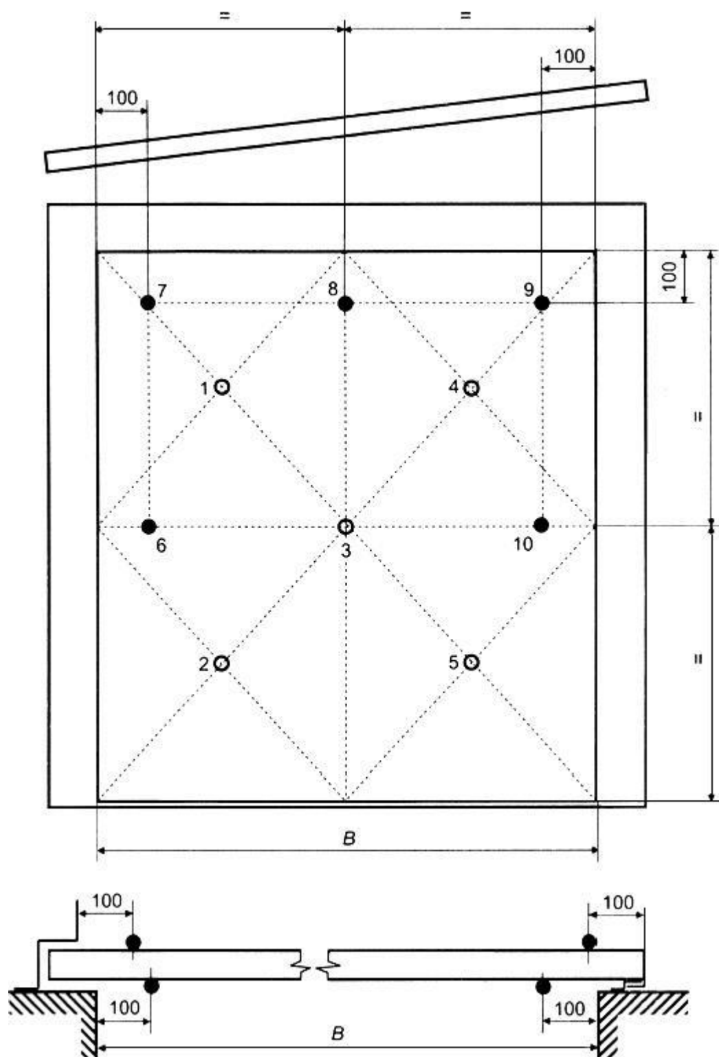
Рисунок 14 - Схема установки термодатчиков на необогреваемой поверхности полотна откатной двери (ворот)
