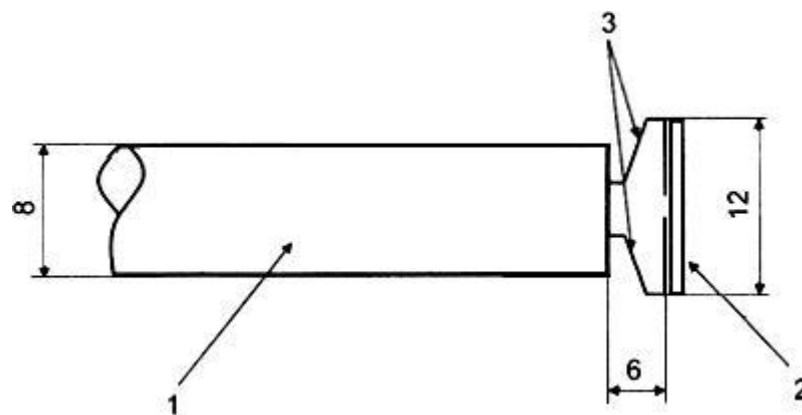
Рисунок 1 - Конструкция переносной термопары
