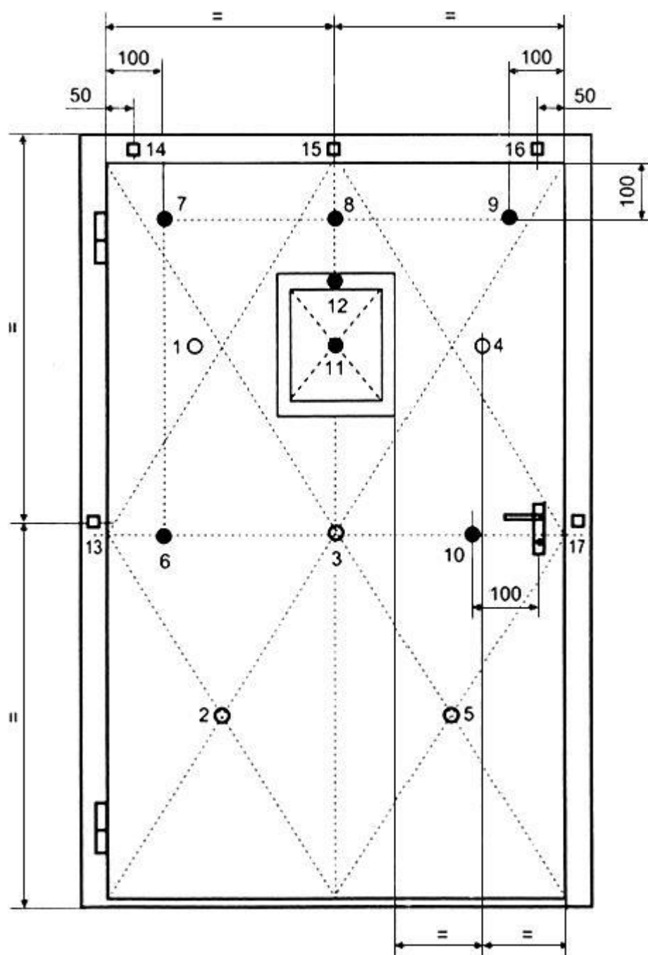
Рисунок 21 - Схема установки термодпар на необогреваемой поверхности распашной однопольной двери с частичным остеклением
