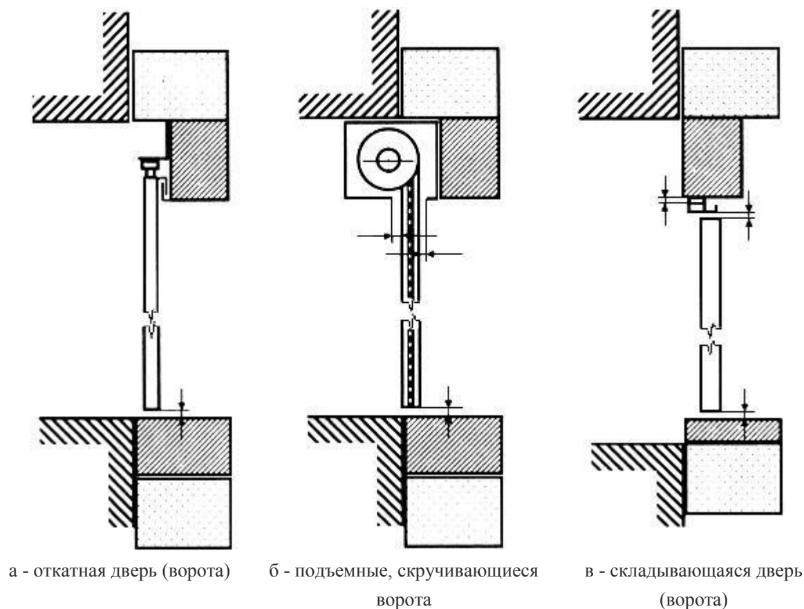
Рисунок 27 - Примеры замеров зазоров (вертикальное сечение)
