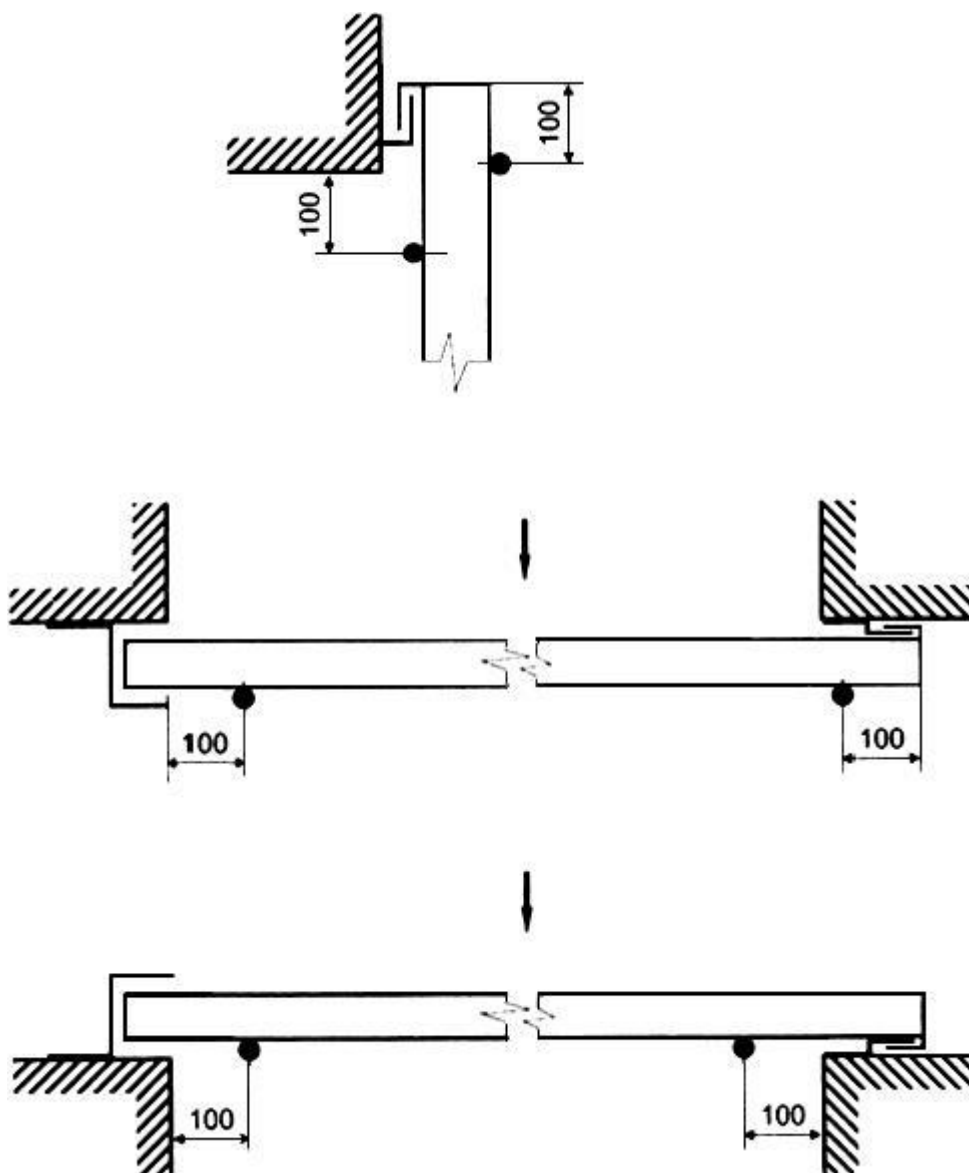
Рисунок 15 - Схема установки термодатчиков на необогреваемой поверхности полотна откатной двери (ворот) в зоне 100 м от его торцевых поверхностей, края, коробки и проема в свету
