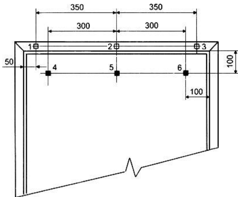
Рисунок 23 - Количество термопар, устанавливаемых в зависимости от ширины полотна (коробки)
