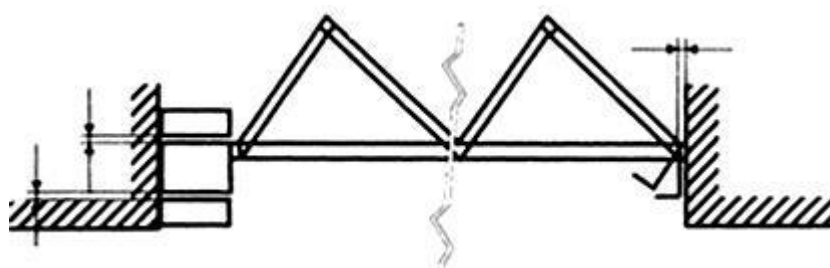
в - складывающаяся дверь (ворота)
